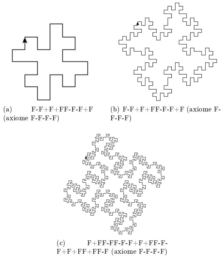
FIGURE 2 – Une autre courbe de Koch
