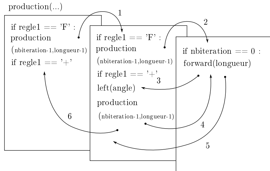
FIGURE 7 – Flocon de Koch récursif.
