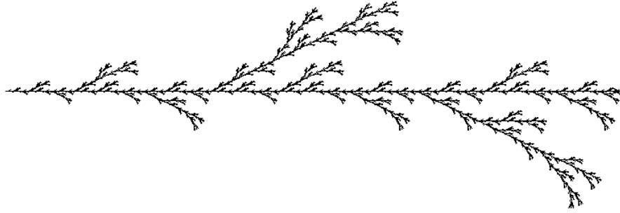
FIGURE 3 – Modélisation d'une plante
