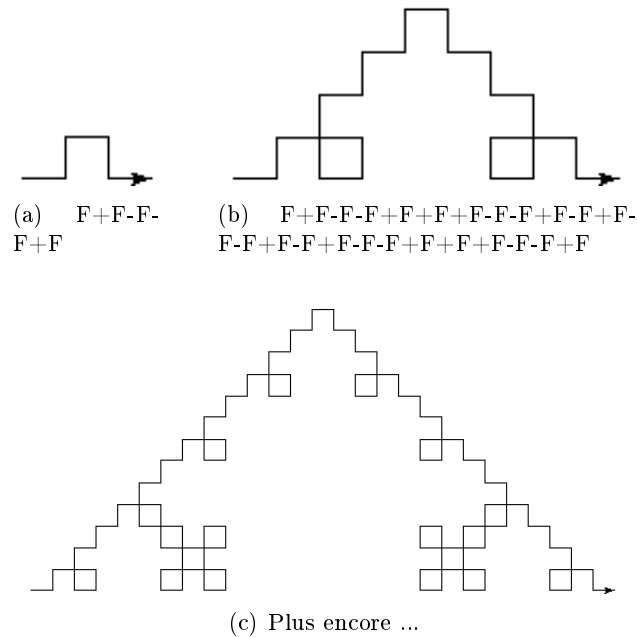
FIGURE 1 – La courbe de Koch
