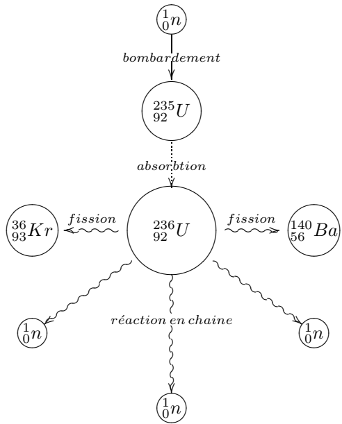
FIG. 1 – Fission de l'uranium
