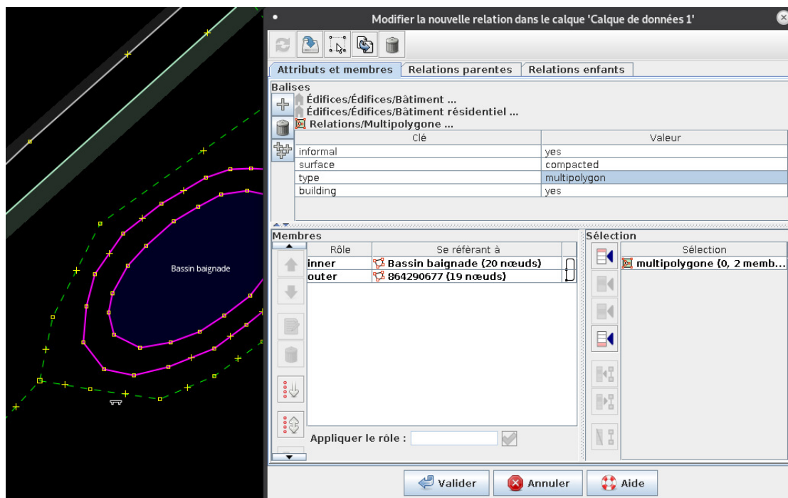
FIGURE 57 – Éditeur de relations de JOSM.
