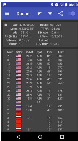
(b) GPSTest
